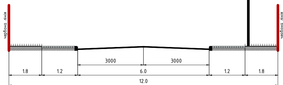
Поперечний профіль вулиці з червоними лініями М 1:100 I-I
