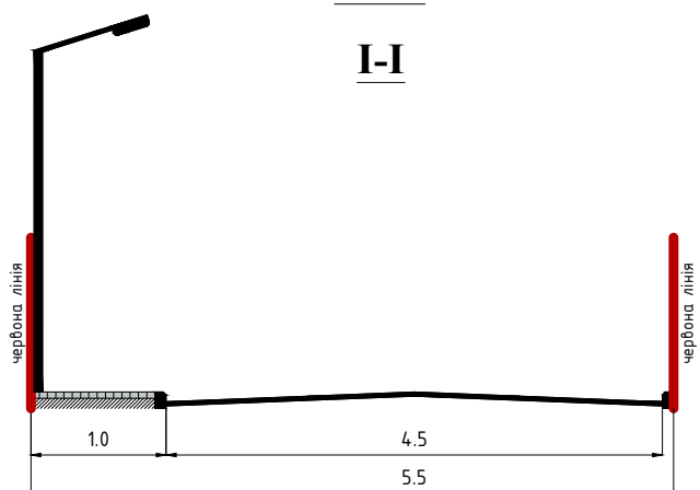
Поперечний профіль вулиці з червоними лініями М 1:100
