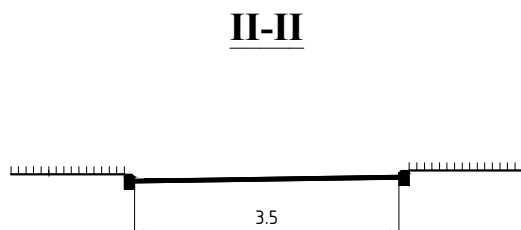
Поперечний профіль проїзду М 1:100
